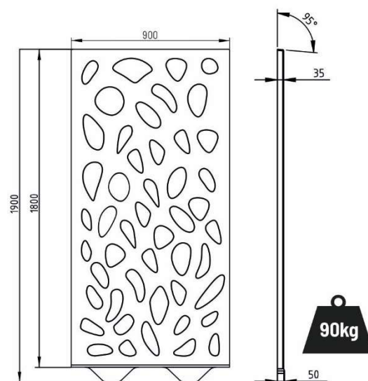
Wymiary techniczne produktu
